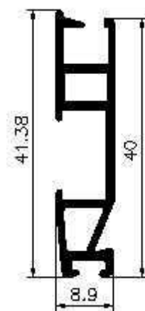
Terminal de mosquiteiro refª 1067
