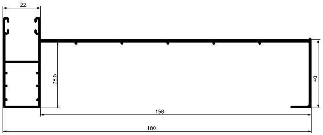
Guia de embutir comando 180 refª 1780
