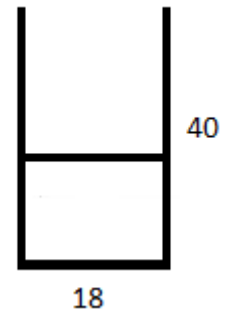
Guia simples de 40 refª 31707
