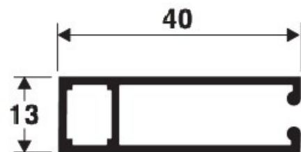
Guia de 40 Rolbox refª 9040
