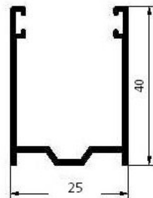
Guia 40 Su refª 1318
