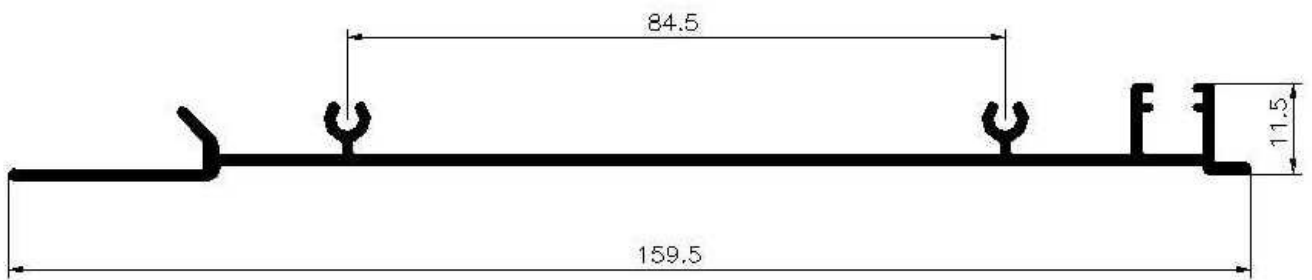
Tampa interior plasbox 155 refª 1167
