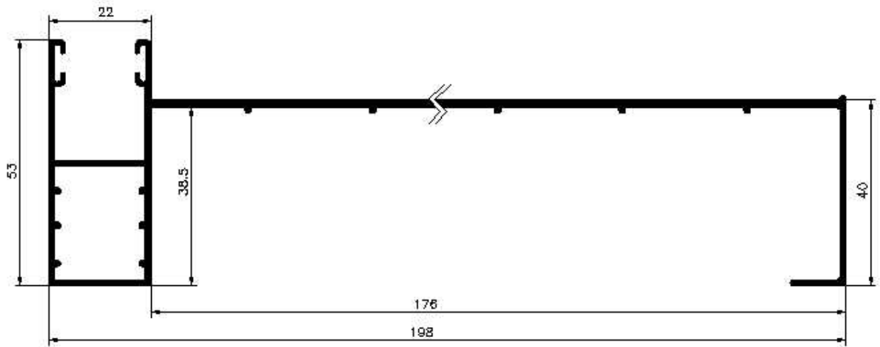
Guia de embutir comando 198 refª 1798
