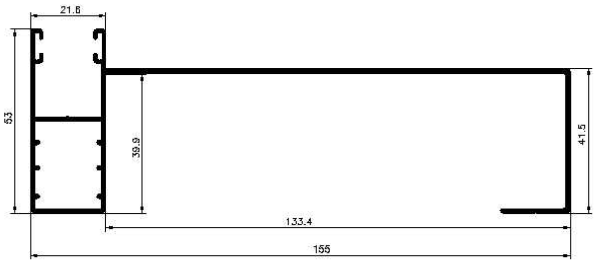
Guia de embutir comando 155 refª 1755
