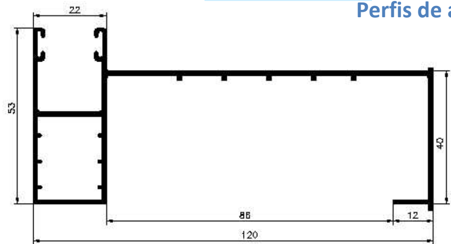
Guia de embutir comando 120 refª 1763
