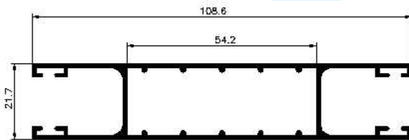
Guia central monobloco refª 1550
