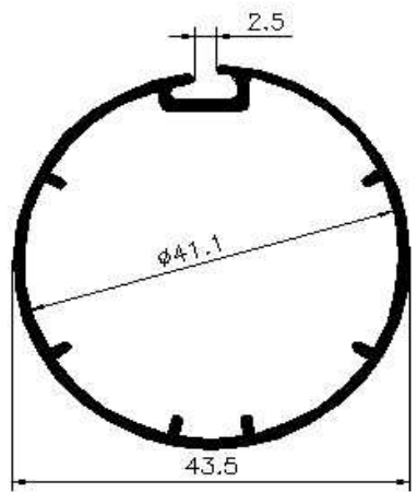
Tubo RI.43 refª 1226
