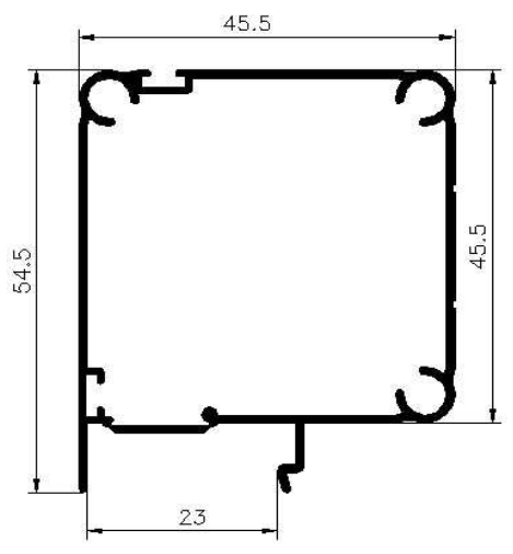
Cofre mosquitoireo de corrente refª 1065
