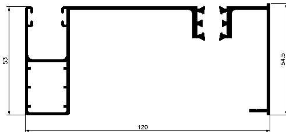
Guia de embutir comando de rutura térmica refª 1720-R
