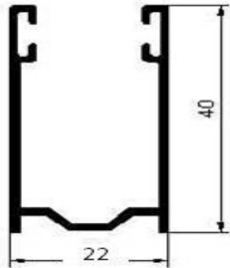
Guia 40 Vd refª 1847
