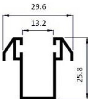
Guia de embutir refª 1495
