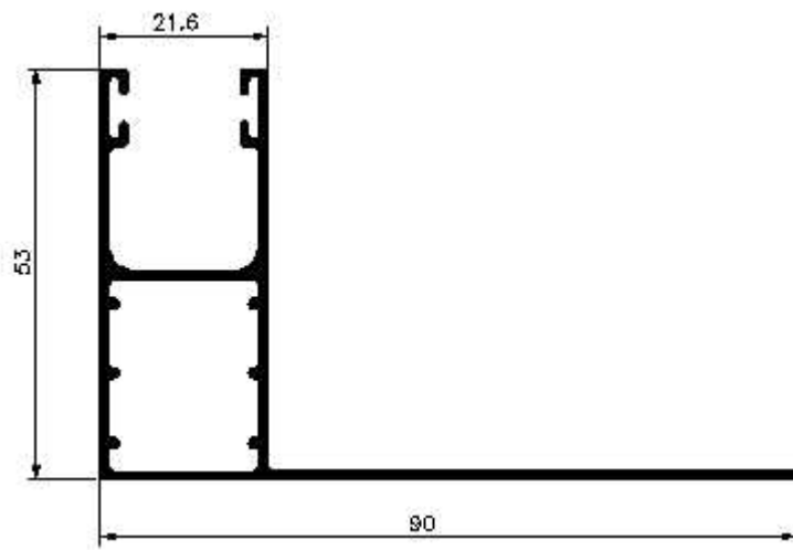
Guia Pala 90 refª 1590
