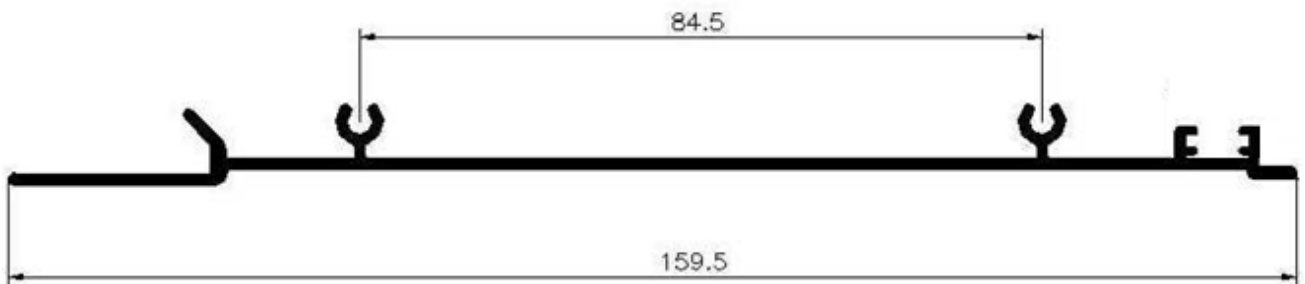
Tampa exterior plasbox 155 refª 4336
