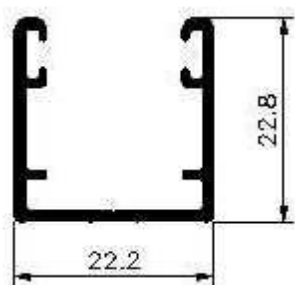
Guia inferior mosquiteiro refª 1069
