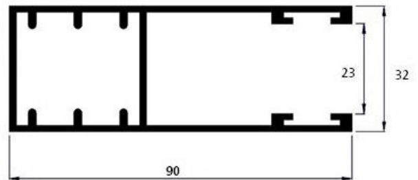
Guia Pf 77 refª 1675
